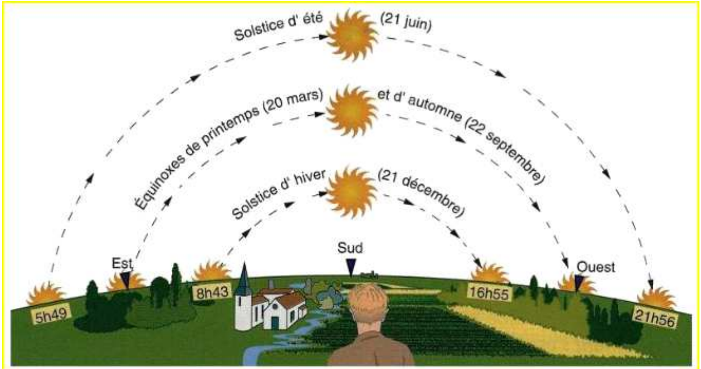
Mouvement apparent du Soleil en fonction des saisons dans les zones tempérées
