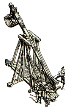
Un trébuchet
