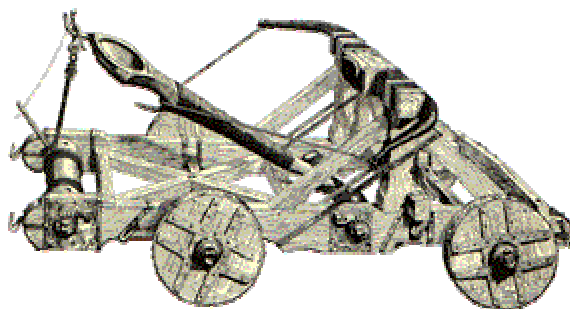
Une catapulte
