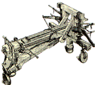
Une baliste
